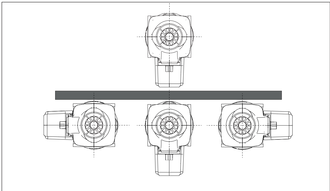
Figura 5. Orientaciones posibles del calefactor
